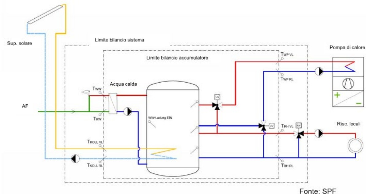
Fig. 1: Sistema verificato (accumulatore e idraulica) con due valvole di commutazione. Lo scambiatore di calore è esemplare e vale anche per scambiatori interni. Il sifone termico non è indicato nello schema.
